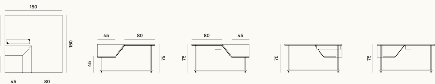
Worktop / Sedia / Chaise CREMOD02
