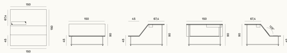
Chaise longue / Sedia / Chaise CREMOD03
