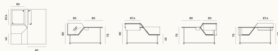
Chaise longue / Sedia / Chaise CREMOD06
