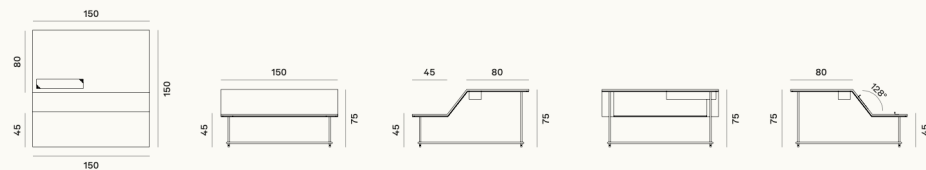
Chaise longue / Sedia / Chaise CREMOD04
